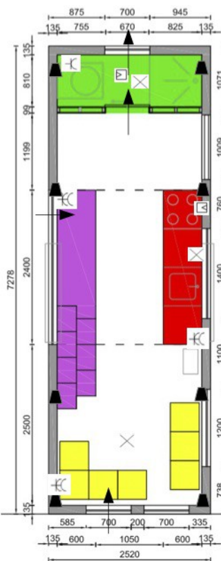
begane grond
