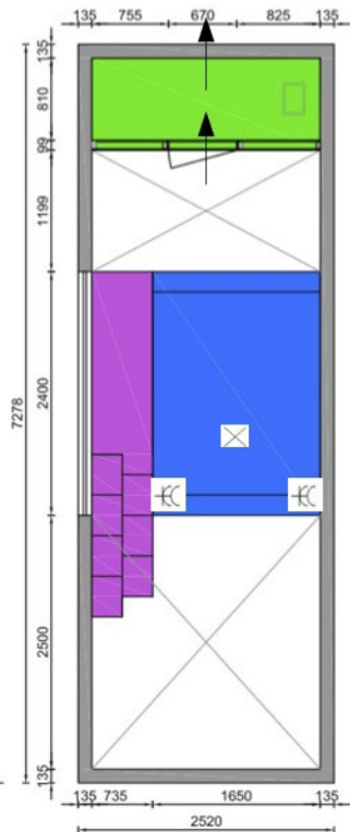
verdieping
