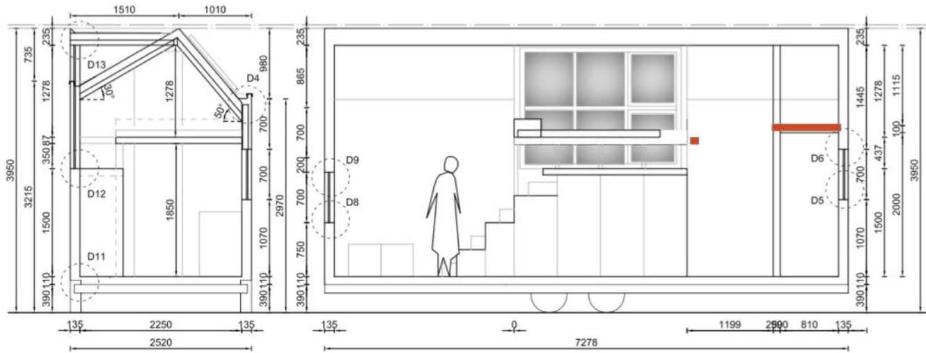
dwarsdoorsnede
