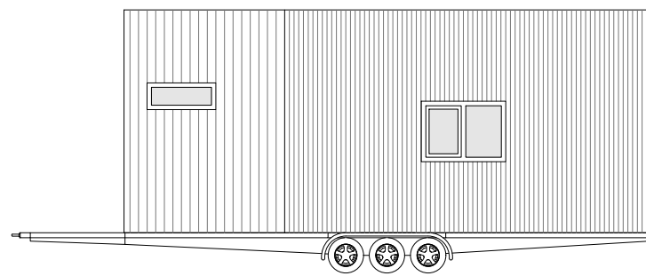
ACHTERGEVEL
