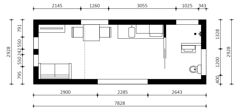
PLATTEGROND
